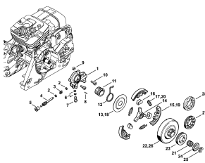
Olejoyé čerpado, spojka
