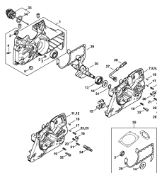
Kliková skříň
