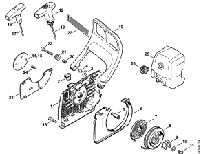
Startovací zařízení
