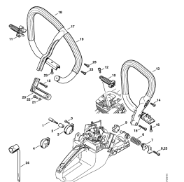
Systém AV, trubka rukojeti
