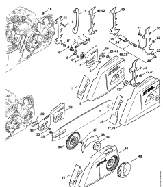
Zařízení pro napínání řetězu
