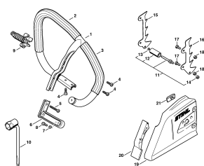
Souprava "Přední trubková rukojeť"
