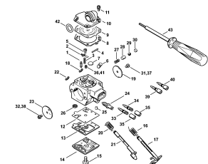
Karburátor HD-34, HD-46
