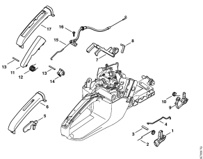
Ovládání plynu
