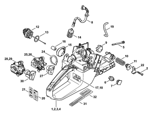
Těleso nádrže
