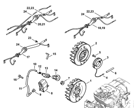
Zapalování, kabelový svazek
