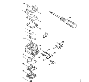
Karburátor C3R-S236, C3R-S279
